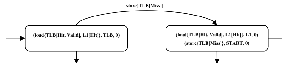
Рис. 4. Фрагмент абстрактной автоматной модели конвейера.
