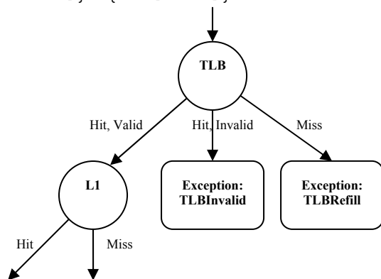
Рис. 3. Фрагмент дерева выполнения инструкций загрузки/сохранения.
