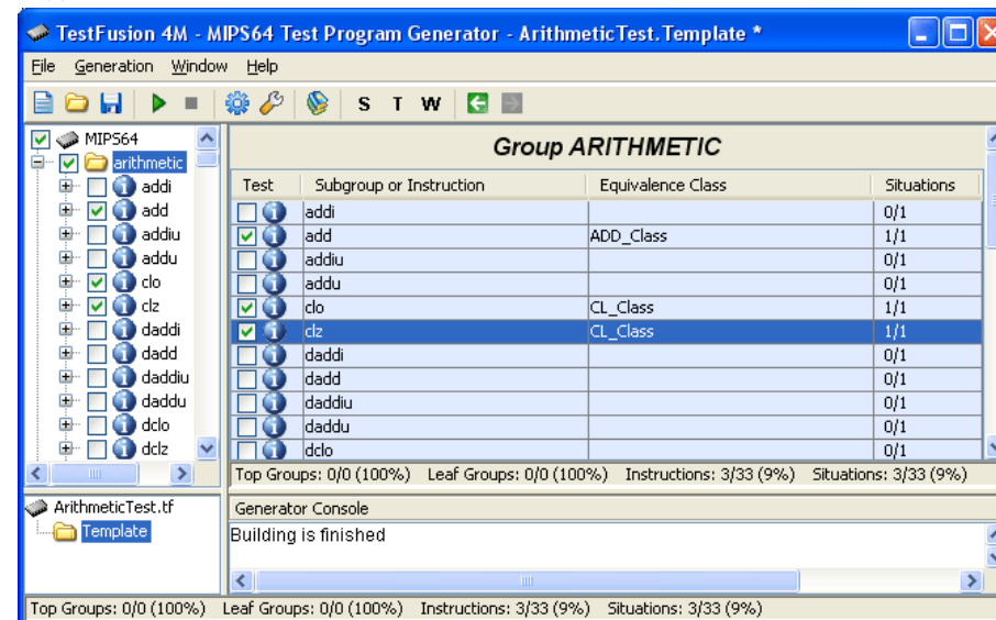
Рис. 2. Графический интерфейс TestFusion 4M.
